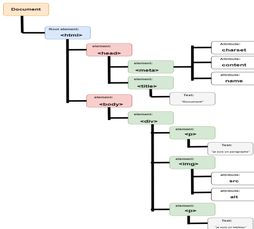
Figure 3: Représentation DOM
